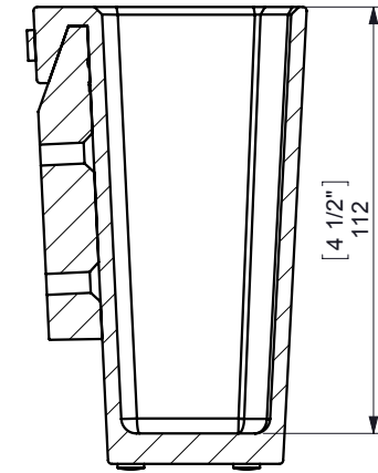
SECCIÓN A-A
