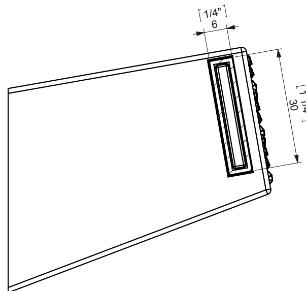
SECCIÓN A-A ESCALA 1 : 1
