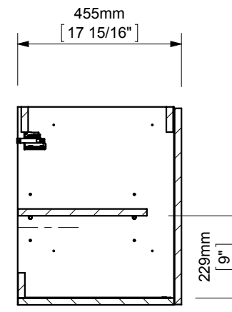
SECCIÓN A-A
