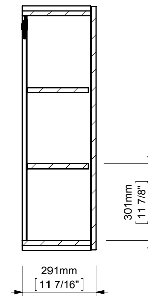
SECCIÓN A-A
