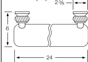
316-0.8 Glass Shelf (TV)
