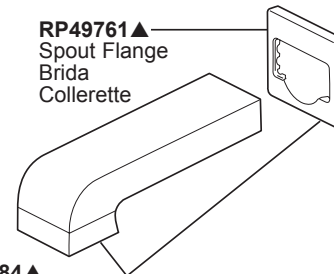
RP64084▲ Tub Spout/Pull-Down Diverter & Flange Tubo de salida para bañera/desviador de halar y brida Bec/avec dérivation sur embout et colerette
