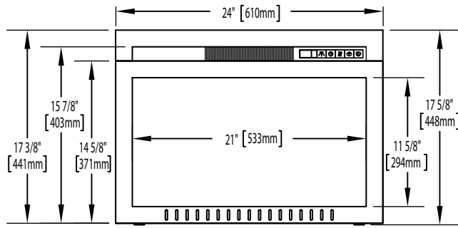
CEFB24H ILLUSTRÉE
