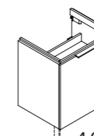
4.0755.1 X: 595 mm Y: 615 mm Z: 455 mm
