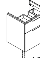
4.0756.6 X: 595 mm Y: 615 mm Z: 455 mm
